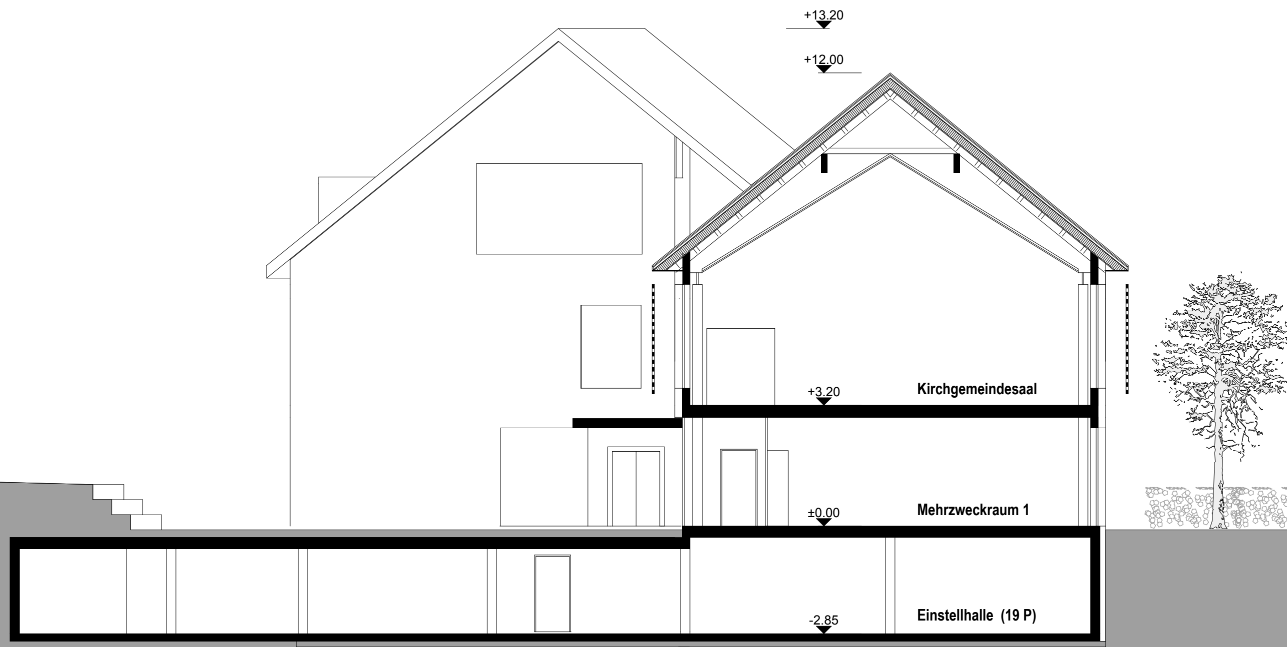
Querschnitt 1
